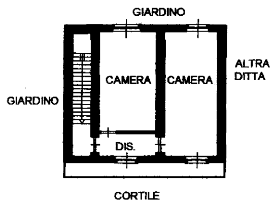
PIANTA PIANO PRIMO H = 2.90 mt.
